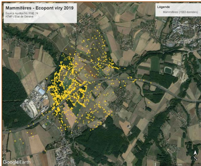
Carte de nos données mammifères collectées lors du suivi faune autour de l'écopont en 2019.
