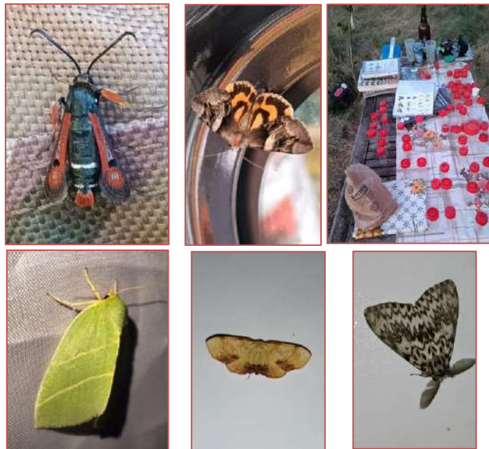
Pyropteron sidiformis , Catocala fulmine , table d'identification, Pseudoips prasinanus , Plagodis dolabraria et Lymantria monacha © Luc Mery
